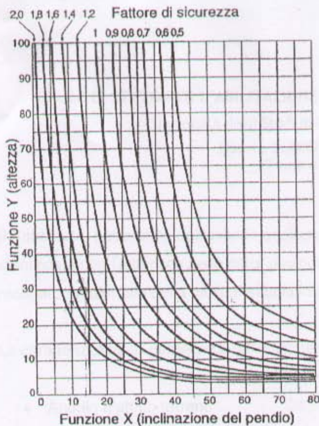
Grafico di progetto e funzioni per superfici di rottura circolari. Le curve indicano i diversi fattori di sicurezza F (Hoeck, 1970).
