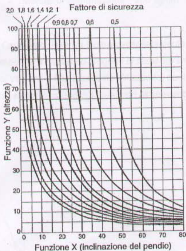
Grafico di progetto e funzioni per superfici di rottura piane. Le curve indicano i diversi fattori di sicurezza F (Hoeck, 1970).
